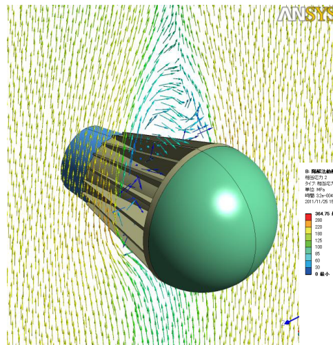
LED 電球周辺の空気の流れ
